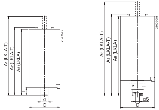
a. 커플링 사용 안 함. a1=d
